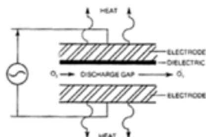
Générateur de décharge corona
